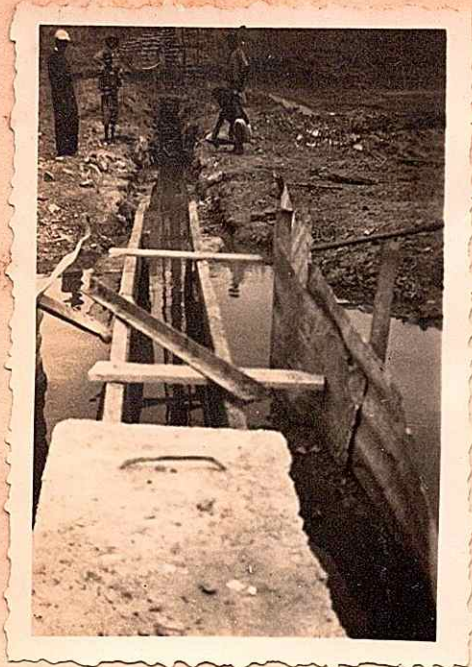
Canal d'amenée en construction du linnigraphe de SEGALA
