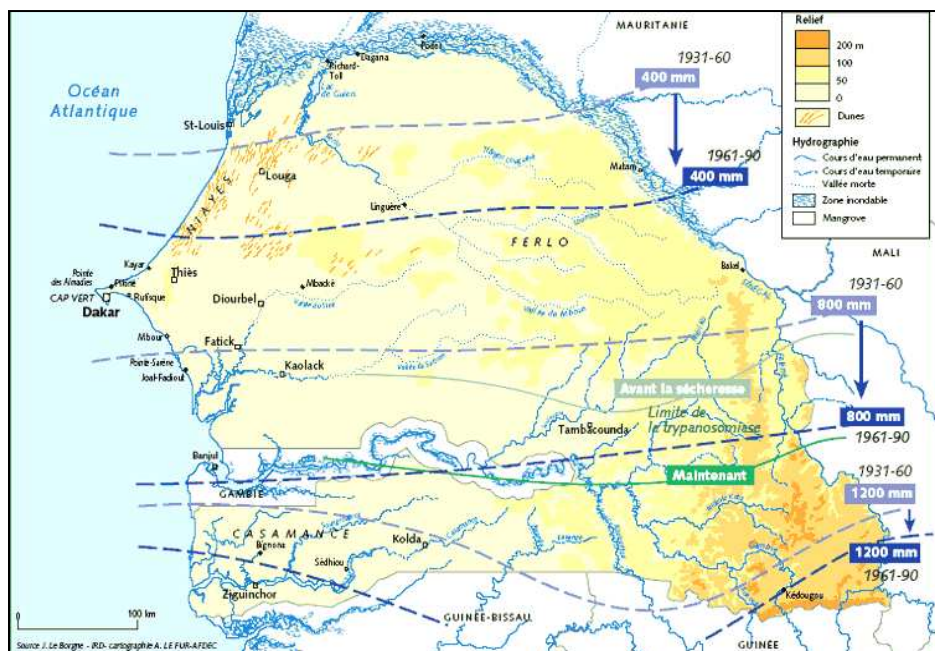
Figure 6 : carte de la translation des isohyètes vers le sud (source : J. Le Borgne, Rapport national sur la biodiversité au Sénégal, 1997)
