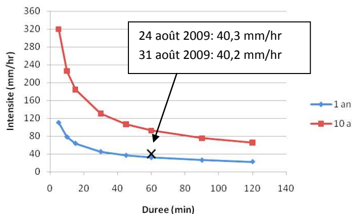
Figure 9 : courbes pluviométriques Intensités-Durée-Fréquence pour Dakar (Yoff)
