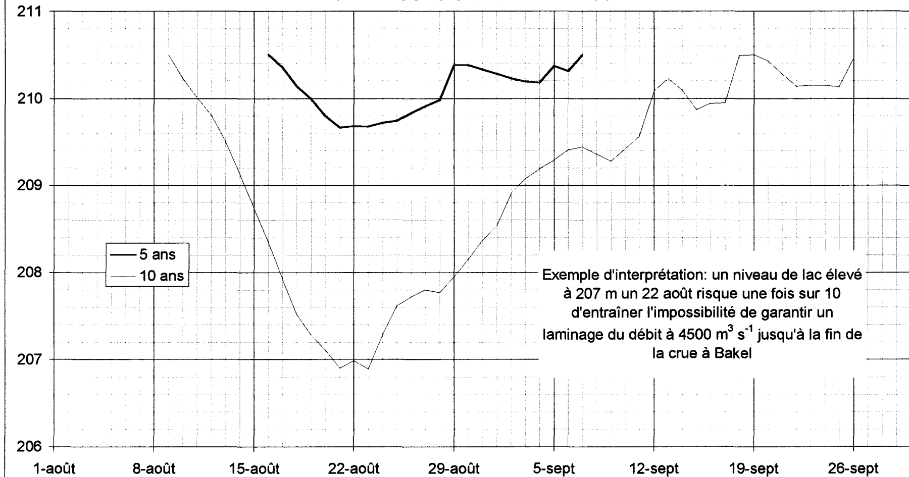
figure 2: cote limite maximale à respecter dans le lac, relative à la revanche nécessaire permettant de laminier le débit du sénégál à Bakel à 4500 \text{ m}^3 \text{ s}^{-1} . Période de référence: 1950-1997
