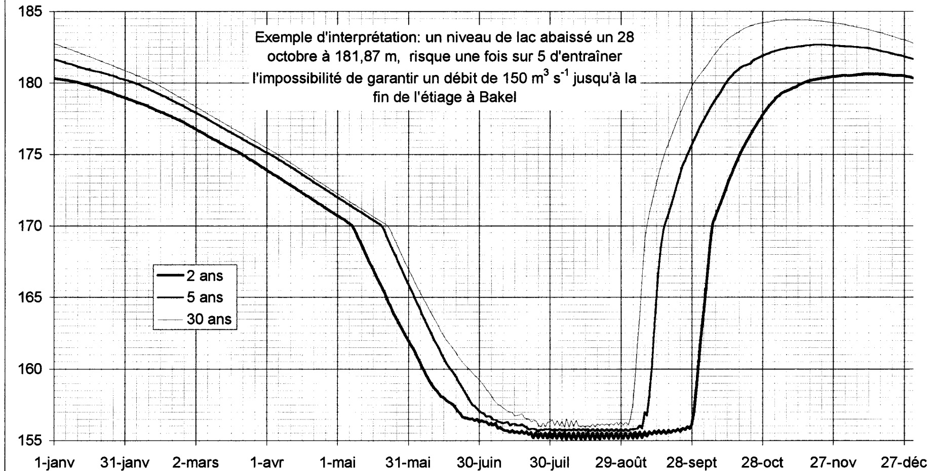
figure 1: cote limite minimale à respecter dans le lac, relative au stock nécessaire pour garantir un débit minimum de 150 \text{ m}^3 \text{ s}^{-1} à Bakel. Période de référence: 1950-1997
