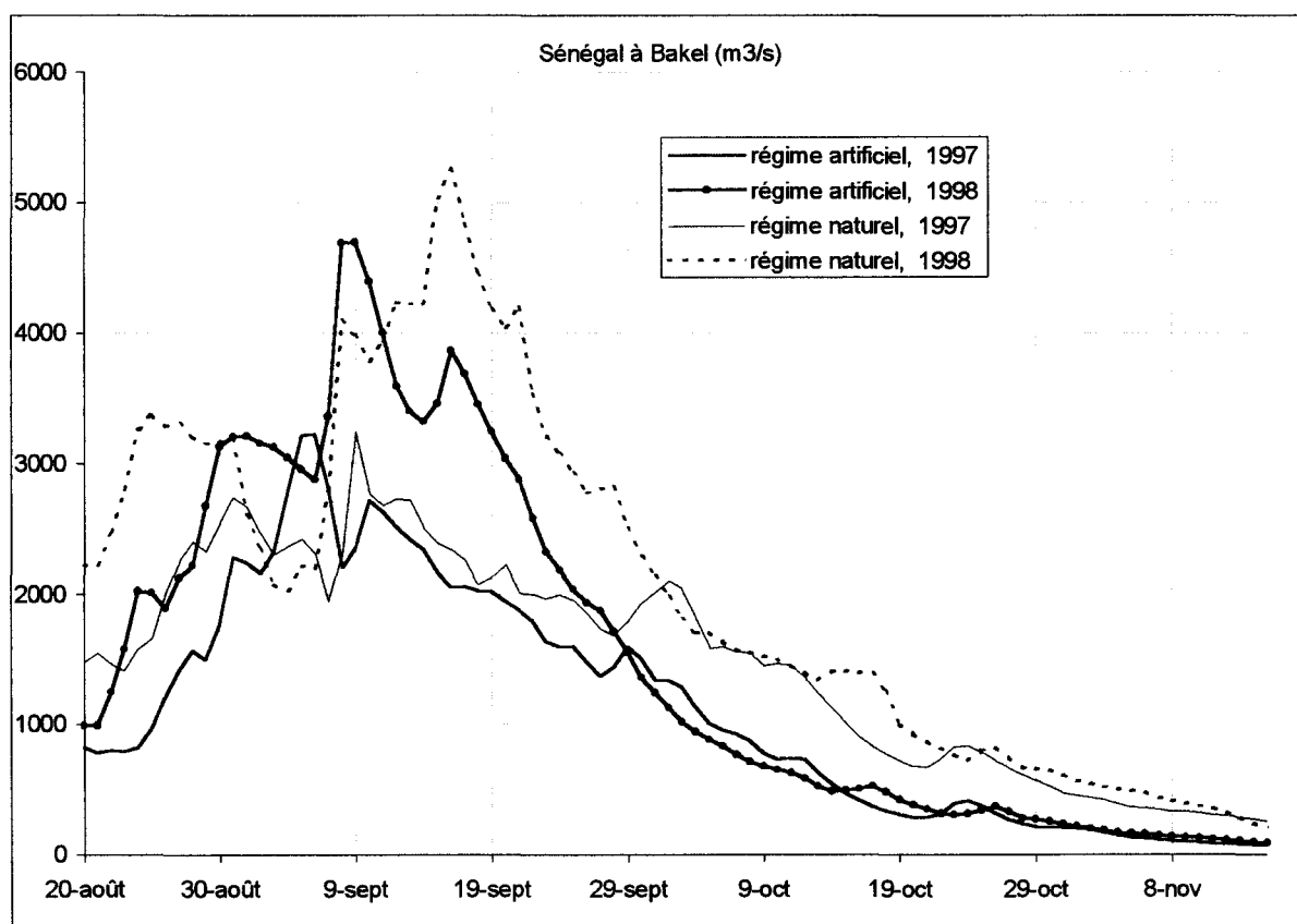
figure 8 : crue du Sénégal à Bakel, 1997 et 1998
