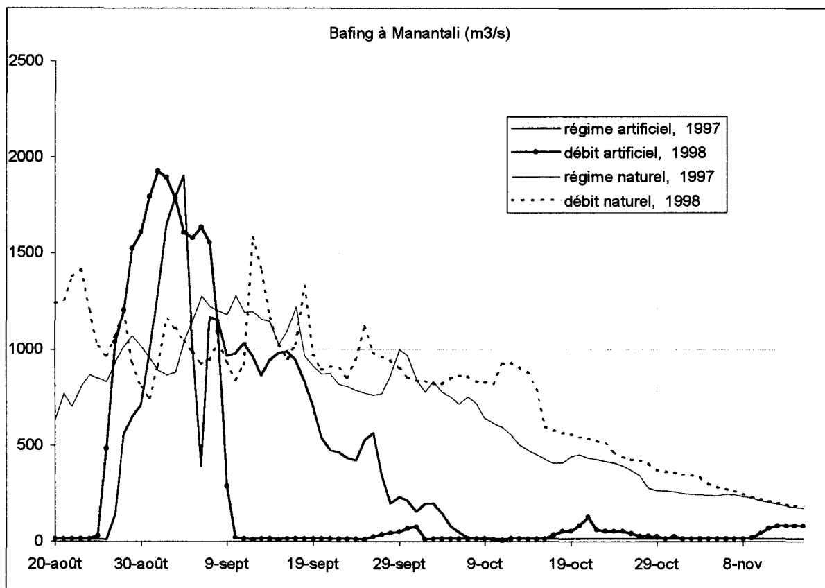
figure 3 : crue du Bafing à Manantali, 1997 et 1998
